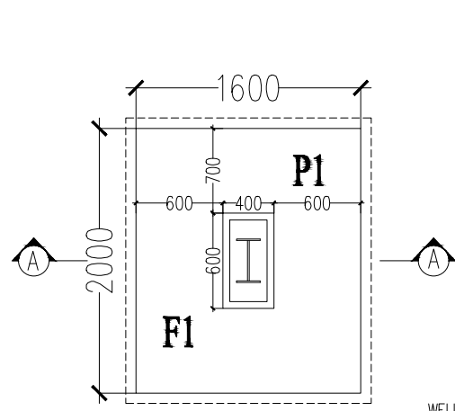
FOOTING PLAN F1
